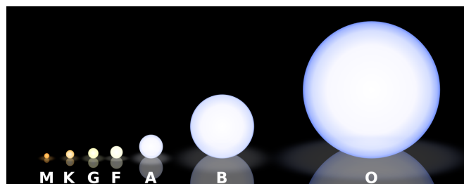
Рис. 12. Звёзды различных спектральных классов [Wikimedia/Rursus]
